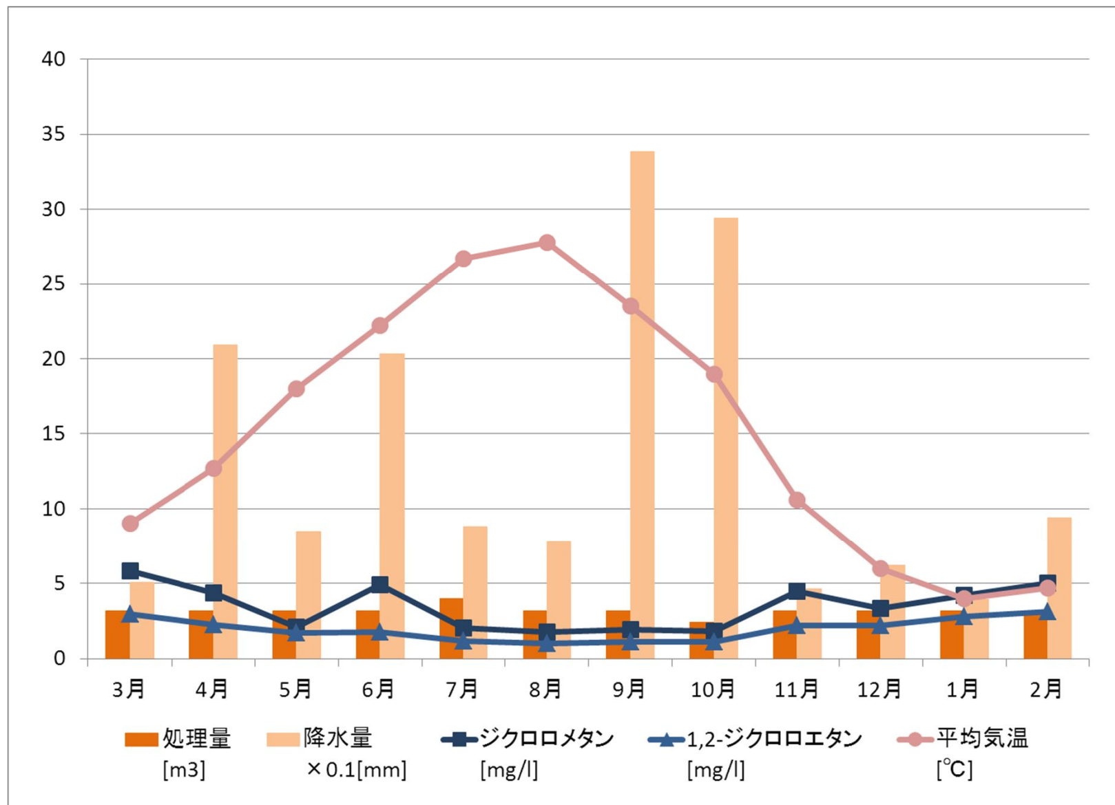
合五工場におけるジクロロメタン濃度、1,2-ジクロロエタン濃度と処理量の推移
