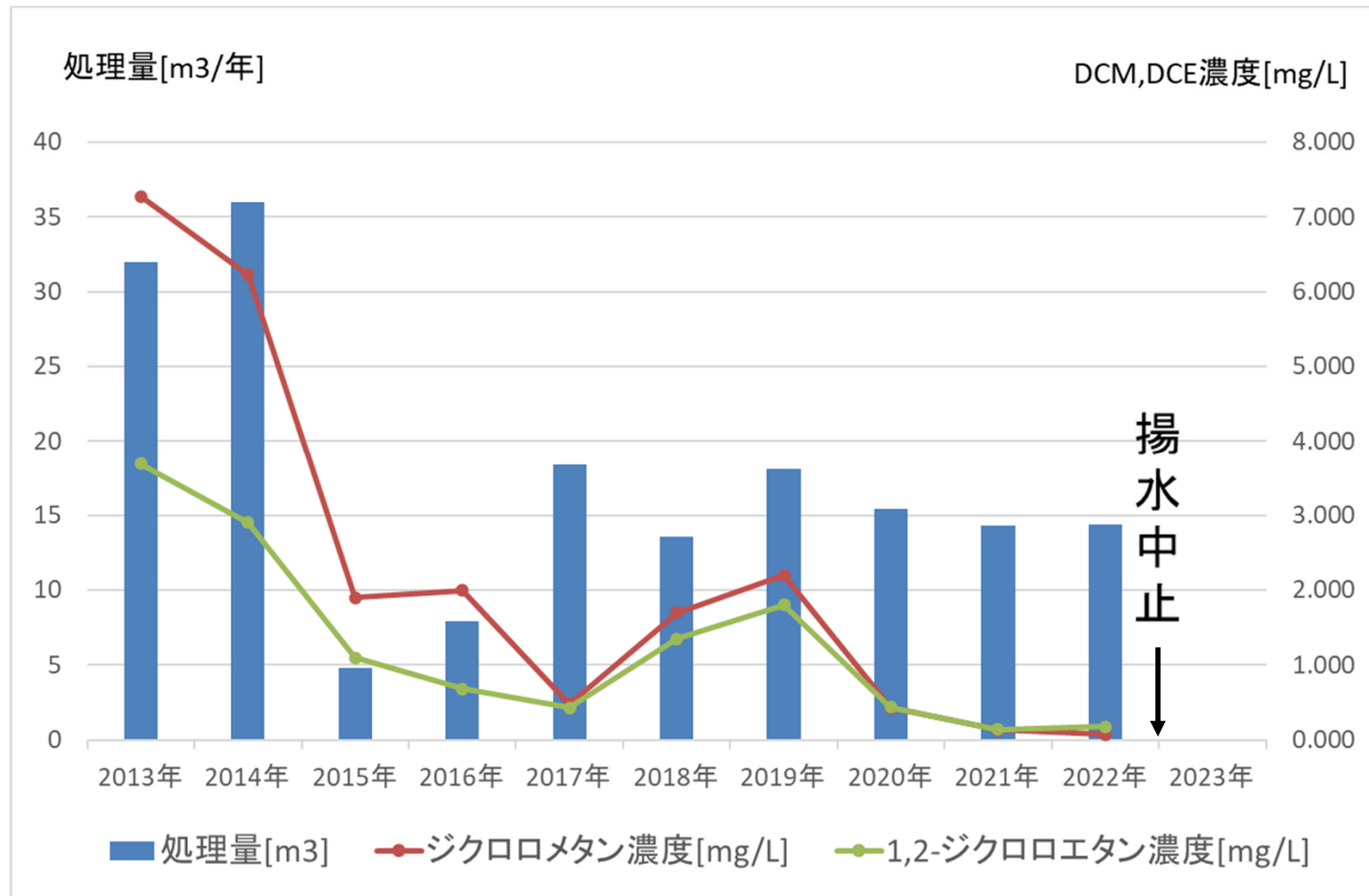
図.合五工場におけるジクロロメタン濃度、1,2-ジクロロエタン濃度と処理量の推移
