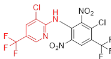
Fluazinam
